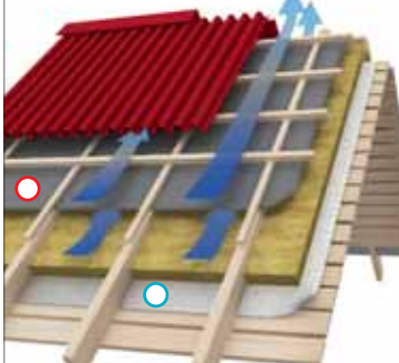
Крыша с двуконтурной вентиляцией
