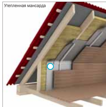
Утепленная мансарда
